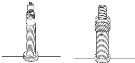
Supapă Sclaverand
